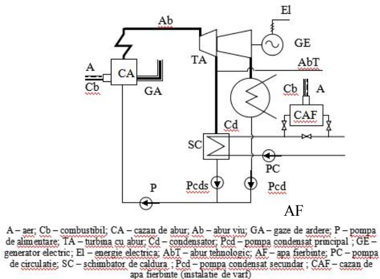
Figura 5.1.3 – Schema de principiu a unei centrale cu turbină cu abur cu condensatie și priză reglabilă
