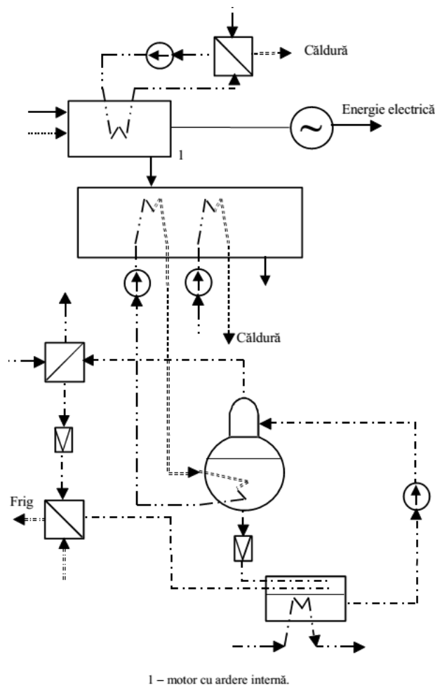
Fig. 5.2.7. Schema de principiu a unei centrale de trigenerare cu motor cu ardere internăcu instalație frigorifică cu absorbție.
