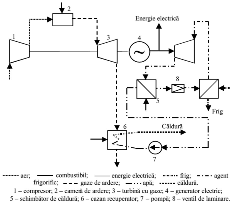
Fig. 5.2.4. Schema de principiu a unei centrale de trigenerare cu turbină cu gazecu instalație frigorifică cu compresie.
