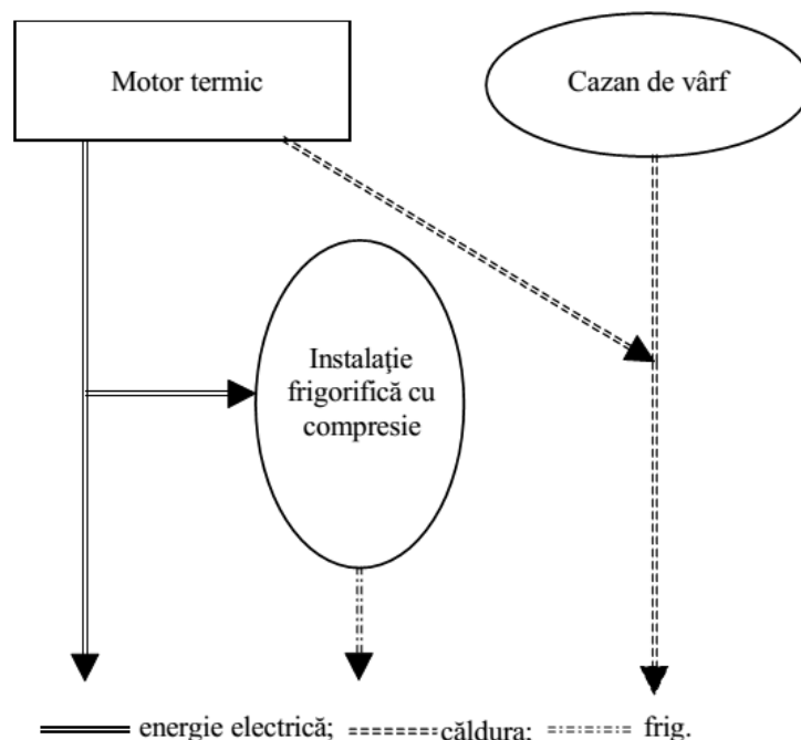
Fig. 5.2.1. Schema de concepție a unei centrale de trigenerare cu instalație frigorifică cu compresie.
