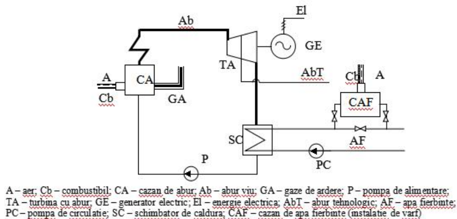
Figura 5.1.2 – Schema de principiu a unei centrale cu turbină cu abur cu contrapresiune și priză reglabilă
