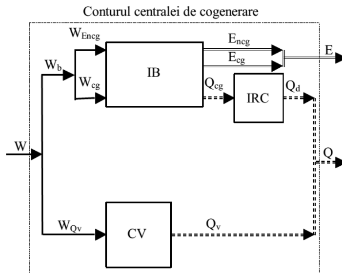
IB – instalație de bază; IRC – instalație de recuperare a căldurii; CV – cazan de vârf
