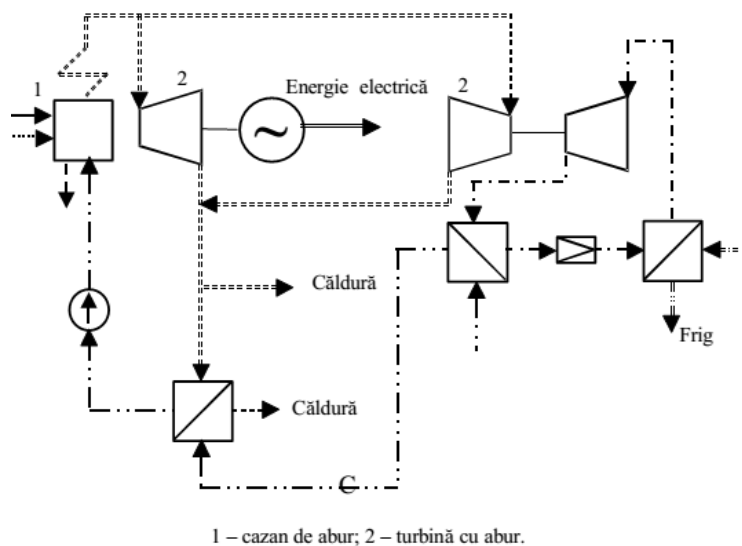
Fig. 5.2.8. Schema de principiu a unei centrale de trigenerare cu turbină cu abur și instalație frigorifică cu compresie.
