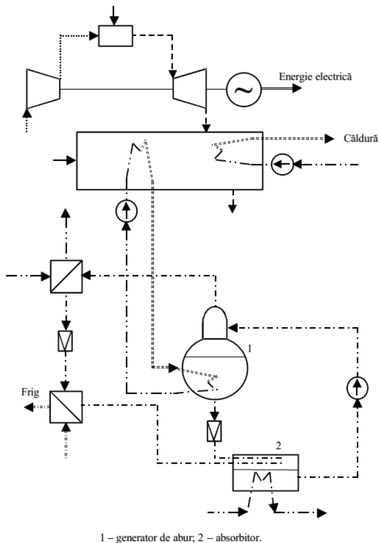
Fig. 5.2.5. Schema de principiu a unei centrale de trigenerare cu turbină cu gazecu instalație frigorifică cu absorbție.
