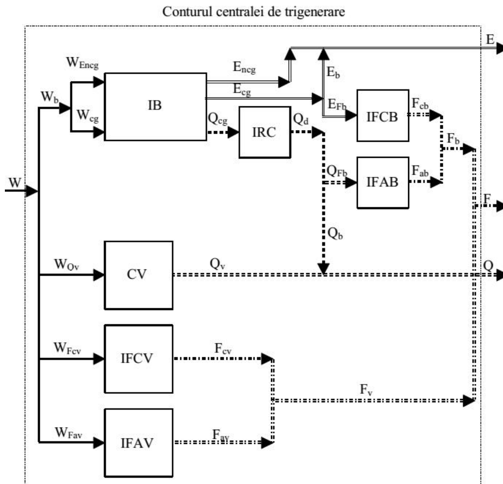
IB – instalație de bază; IRC – instalație de recuperare a căldurii; CV – cazan de vârf; IFCB – instalație frigorifică cu compresie de bază; IFAB – instalație frigorifică cu absorbție de bază; IFCV – instalație frigorifică cu compresie de vârf; IFAV – instalație frigorifică cu absorbție de vârf
