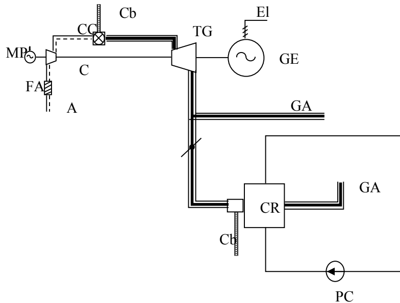
A – aer; FA – filtru de aer ; C – compresor; CC – cameră de combustie; Cb – combustibil; MP – mo gaze; GE – generator electric; El – energie electrica; CR – cazan recuperator; PC – pompă de
