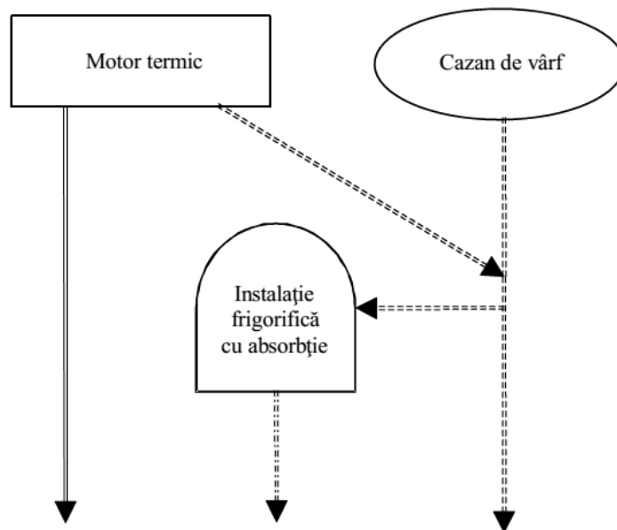
Fig. 5.2.2. Schema de concepție a unei centrale de trigenerare cu instalație frigorifică cu absorbție.
