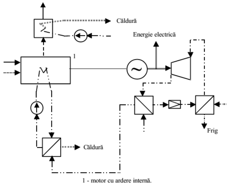
Fig. 5.2.6. Schema de principiu a unei centrale de trigenerare cu motor cu ardere internăcu instalație frigorifică cu compresie.
