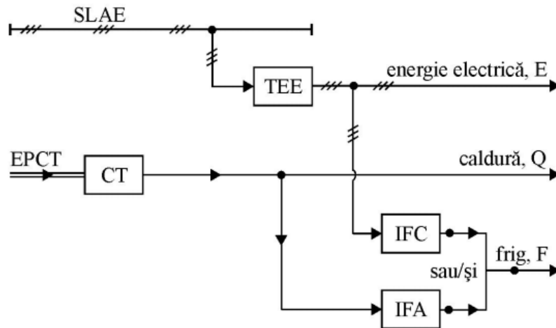
Fig. 5.3.1. Schema de principiu a alimentării separate cu energie electrică, frig și căldură: SLAE – sistemul local de alimentare cu energie electrică; TEE – transformator de energie electrică
